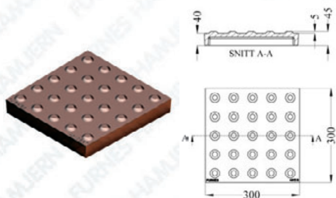
Varselindikator 300x300
