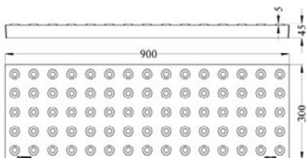
Varselindikator 300x900
